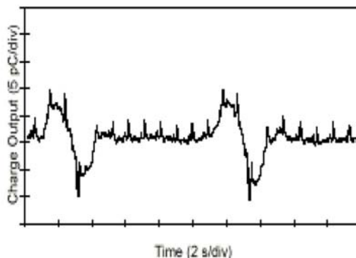
图2 放在垫子和铺有地毯的地面之间时的响应
